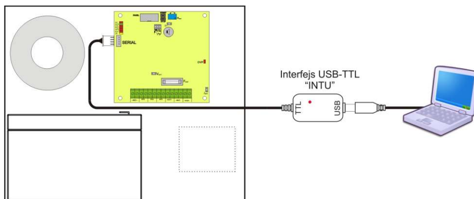
Komunikacja USB-TTL z wykorzystaniem interfejsu USB-TTL „INTU”.
