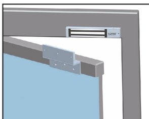
Montaż z uchwytem BK-600WZL2
