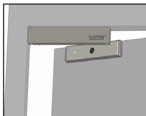
Montaż standardowy / z uchwytem BK-600I
