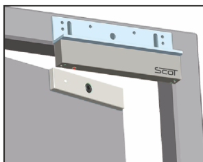
Montaż z uchwytem BK-600WL2
